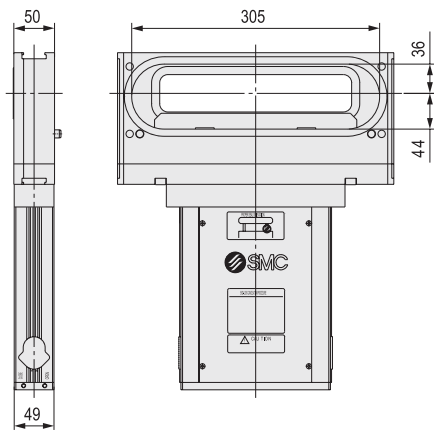
Корпусной тип, Half MESK, XGT223
