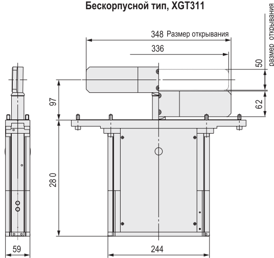
Бескорпусной тип, XGT311
