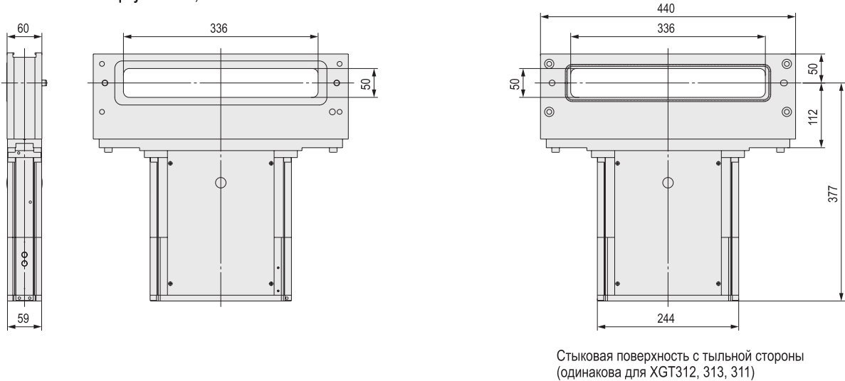
Корпусной тип, XGT312
