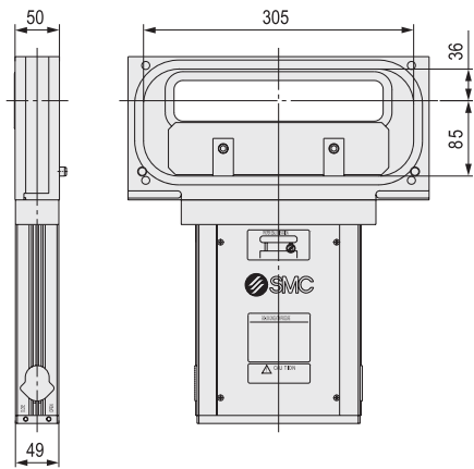
Корпусной тип Full MESK, XGT224
