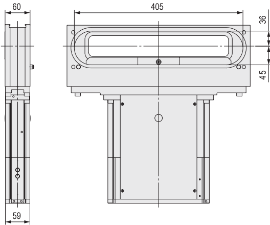
Корпусной тип Half MESK, XGT313
